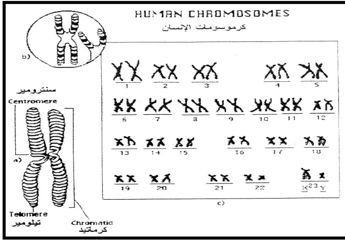
الشكل رقم (٢) كروموسومات الإنسان
