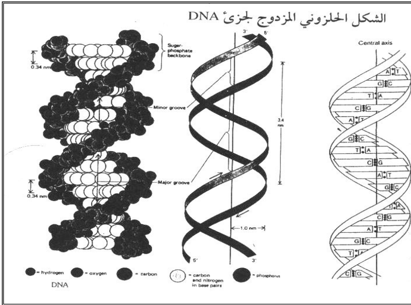
الشكل رقم (٣) الشكل الحلزوني المزدوج لجزء DNA
